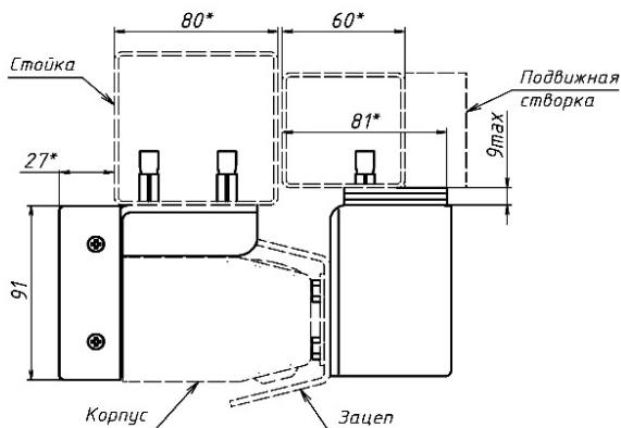
Рисунок 2 (размеры со звездочкой справочные)
