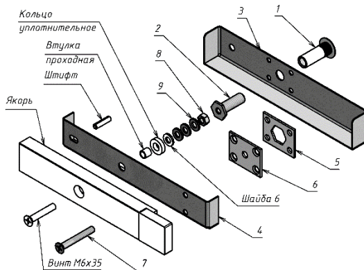
Рисунок 1 – Комплект поставки
