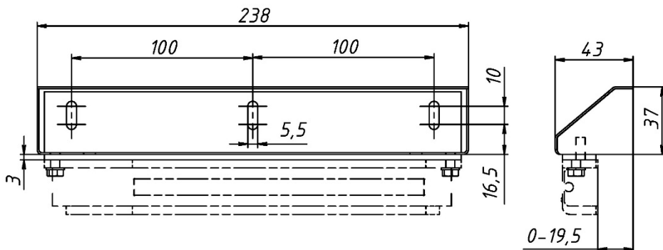
Рисунок 2 – Габаритный чертеж
