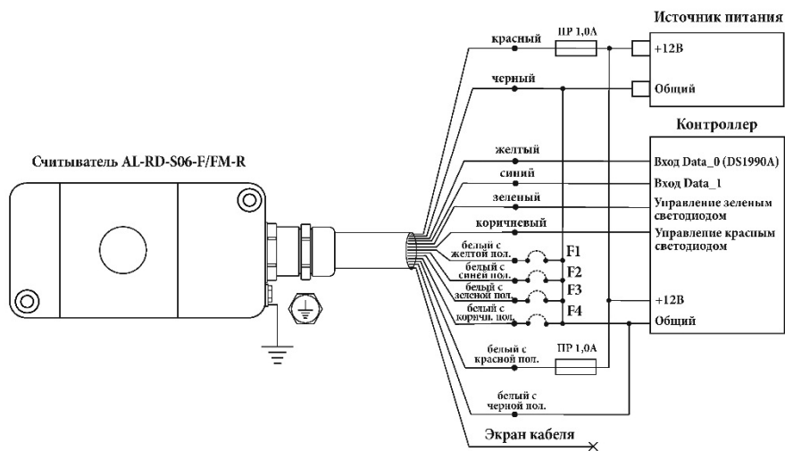
Рисунок 4 – Схема подключения счетчика AL-RD-S06-F/FM-R к контроллеру СКУД с питанием счетчика и нагревателя от одного источника питания.
