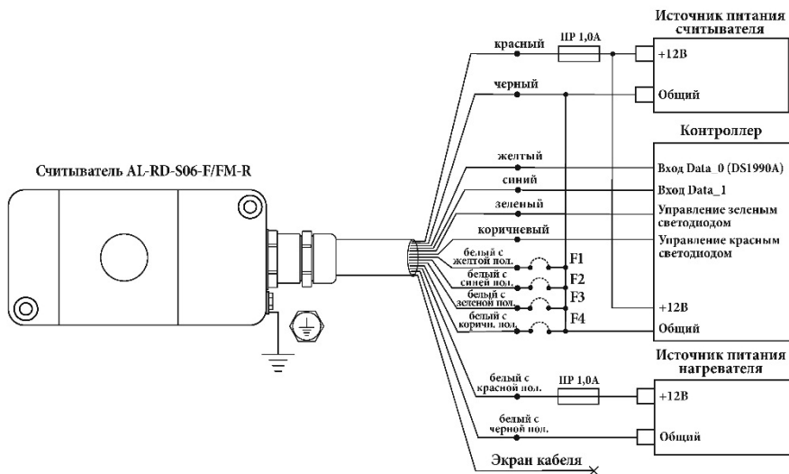
Рисунок 3 – Схема подключения счетчика AL-RD-S06-F/FM-R к контроллеру СКУД с раздельным питанием счетчика и нагревателя.
