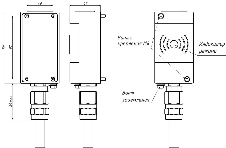
Рисунок 1 - Габаритно-установочные размеры считывателя AL-RD-S06-F/N-R
