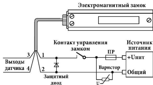
Вариант исполнения со встроенным датчиком Холла (-Н) или герконом (-G)
