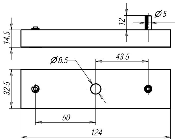
Рисунок 7 - Якорь
