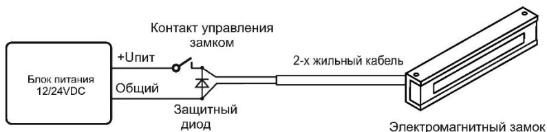
Рисунок 8 – Схема подключения замка
